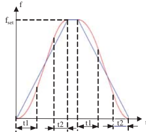
图6-13 S曲线加减速A示意图
