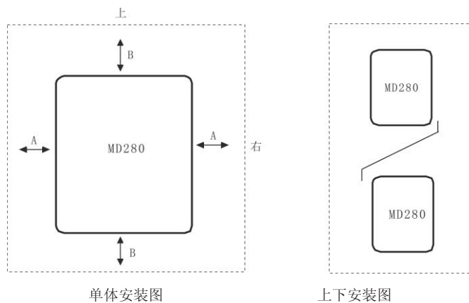
图3-1 MD280变频器安装示意图
