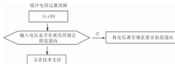
图8-7 缓冲电阻过载故障（Err08）
