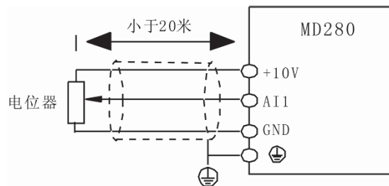
图3-9 模拟量输入端子接线示意图
