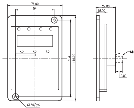
图2-8 外引键盘外型尺寸示意图
