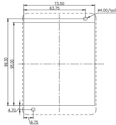
图2-9 外引键盘安装开孔示意图
