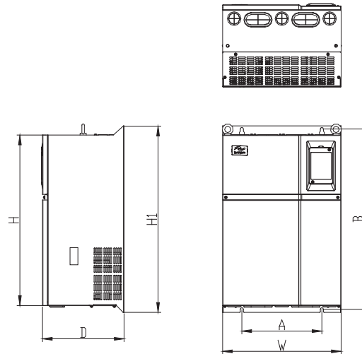
图2-7 MD280NT18.5G/22P~MD280NT400G/450P外型尺寸及安装尺寸示意图
