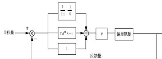
图6-20过程PID原理框图
