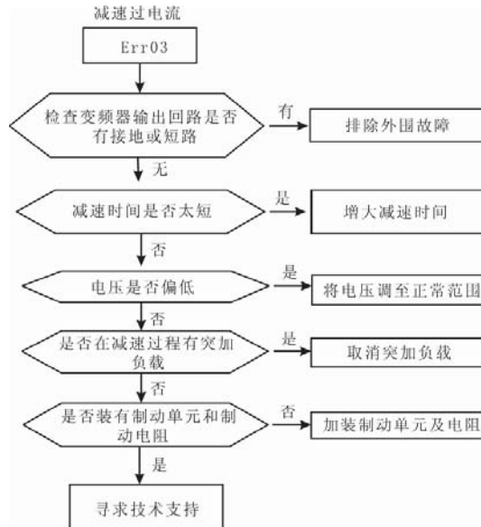
图8-2减速过电流 (Err03)
