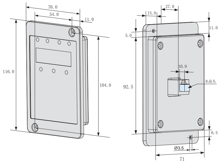
图 2-8 外引键盘的外型尺寸 (单位: mm)
