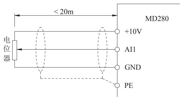
图 3-24 模拟量输入端子接线示意图
