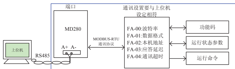
图 3-31 变频器串行通讯的使用
