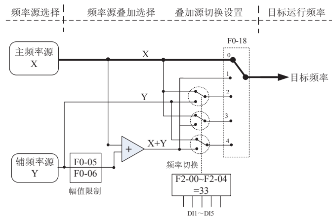
图 5-19 目标频率与主辅频率源的关系
