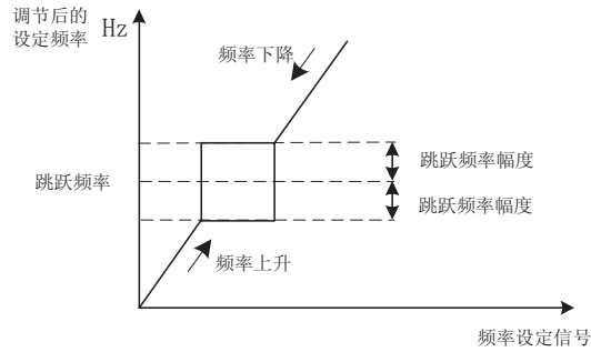
图 5-39 跳频示意图
