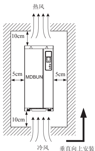
图 2-13 MDBUN 系列制动单元的安装间距
