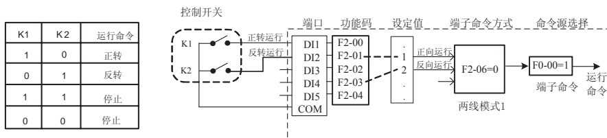
图 5-5 两线式模式 1
