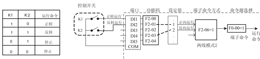
图 5-6 两线式模式 2
