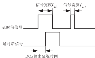
图 5-31 DOx 输出延迟时间示意图
