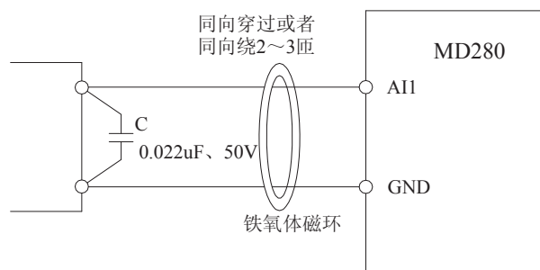
图 3-25 模拟量输入端子处理接线图
