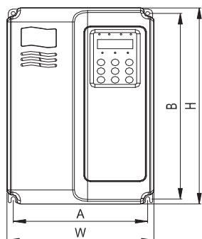
图 2-4 MD280NS0.4GB ~ MD280NT15GB/18.5PB 外型尺寸及安装尺寸示意图
