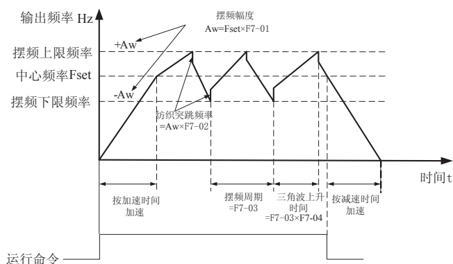
图 5-44 摆频运行示意图
