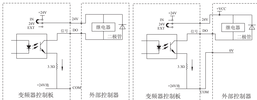
图 3-28 使用内部电源（左）、使用外部电源（右）的 DO 输出接线方式
