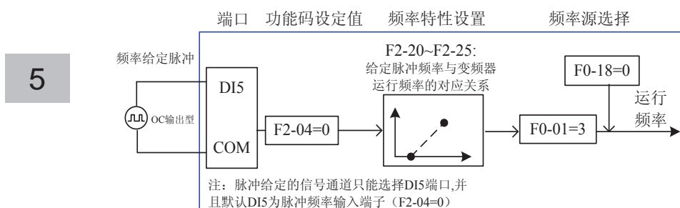
图 5-12 脉冲给定频率功能码设置
