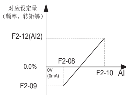
图 3-29 模拟给定与设定量的对应关系
