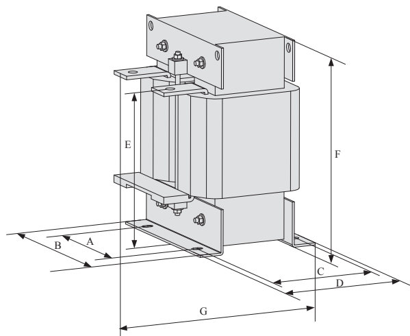
图 2-10 外置电抗器尺寸示意图
