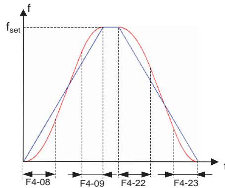
图 5-24 S 曲线加减速 C 示意图
