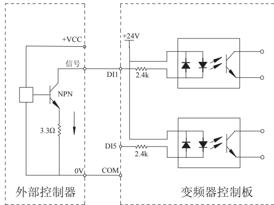
图 3-26 DI 输入接线方式
