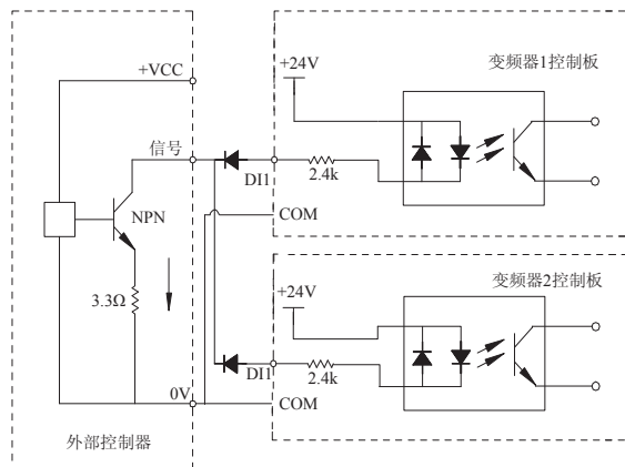
图 3-27 DI 输入接线方式（不同变频器的 DI 端子不能并接使用）
