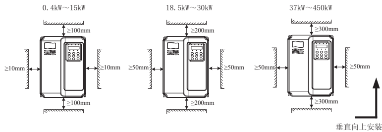
图 3-1 MD280 变频器安装空间要求
