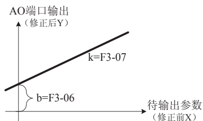
图 3-30 运行参数修正特性曲线
