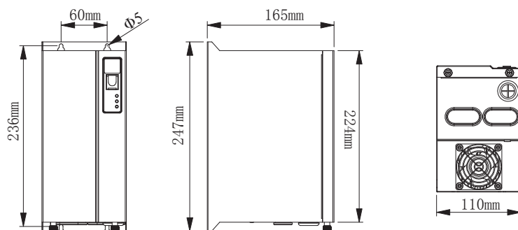
图 2-12 MDBUN 系列制动单元外型尺寸图
