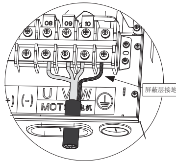
图 6-4 屏蔽电缆接地示意图
