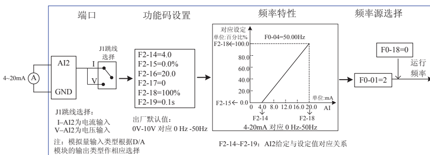
图 5-30 AI2 电流型输入给定频率功能码设置
