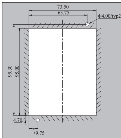
图 2-9 外引键盘安装开孔示意图
