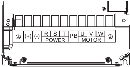
图 3-19 MD280NT7.5GB/11PB- MD280NT 15GB/18.5PB 接线端子分布图
