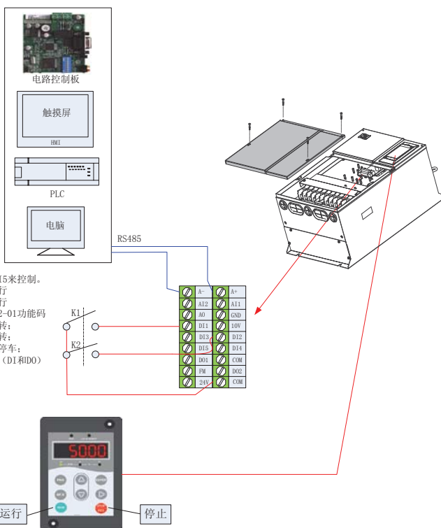
图 5-4 启停命令源说明
