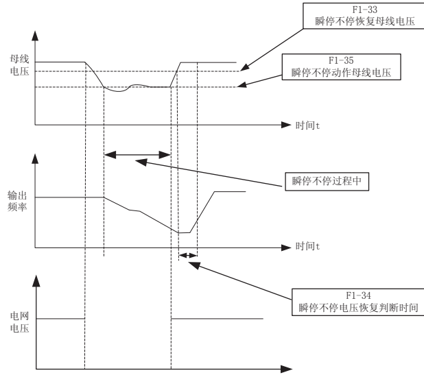
图 5-37 瞬停不停过程示意图
